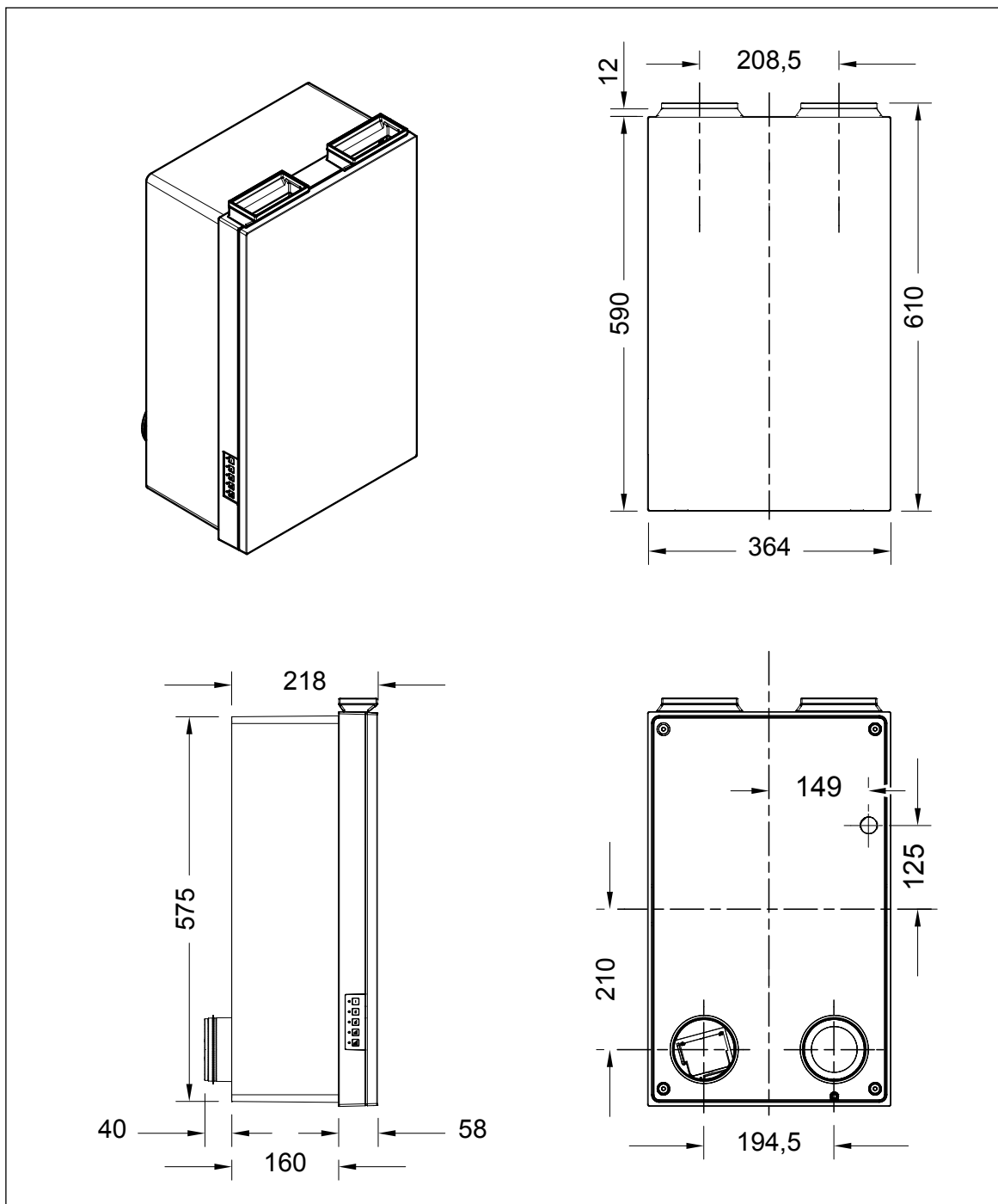
Рис. 10: вентустановка M-WRG-II с адаптером воздуховода для настенного и внутристенного монтажа U 2 , размеры в миллиметрах
