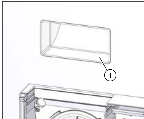
Рис. 41: очистить воздуховод
